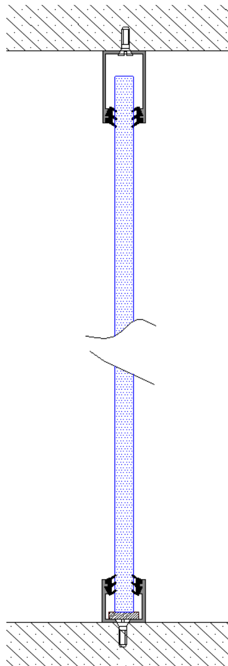
soloVETRO einscheibig Schnitte
